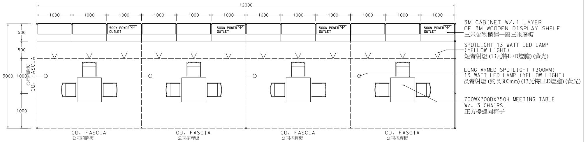
PLAN 平面圖
