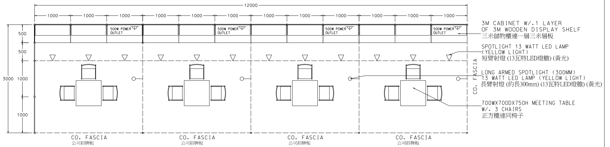
PLAN 平面圖
