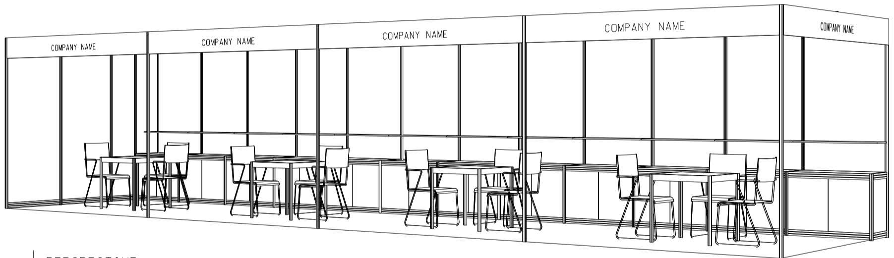
PERSPECTIVE 透視圖
