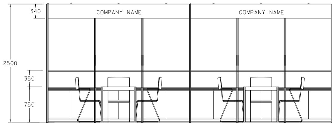
ELEVATION 正面圖
