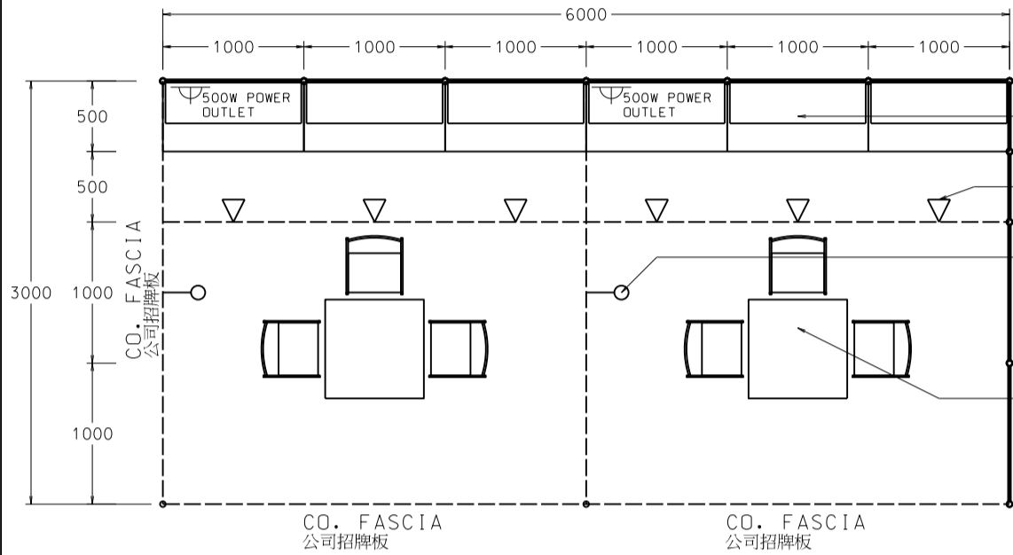
PLAN 平面圖
