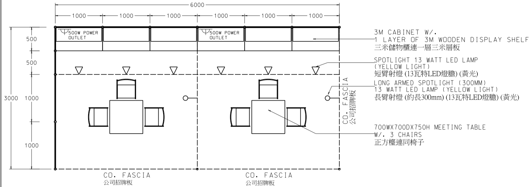
PLAN 平面圖
