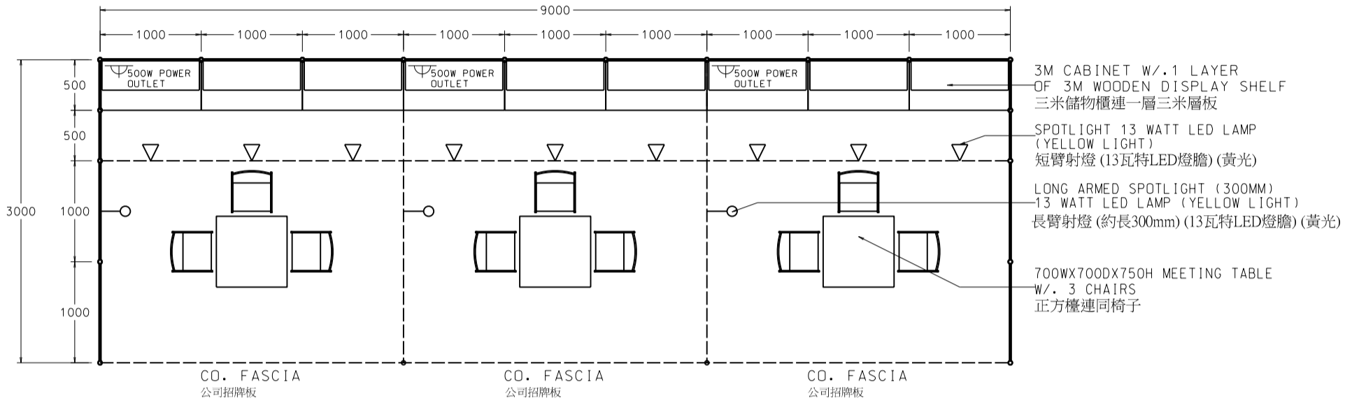
PLAN 平面圖
