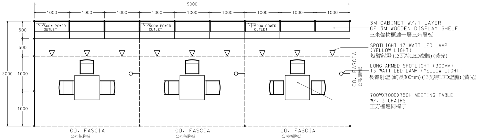
PLAN 平面圖
