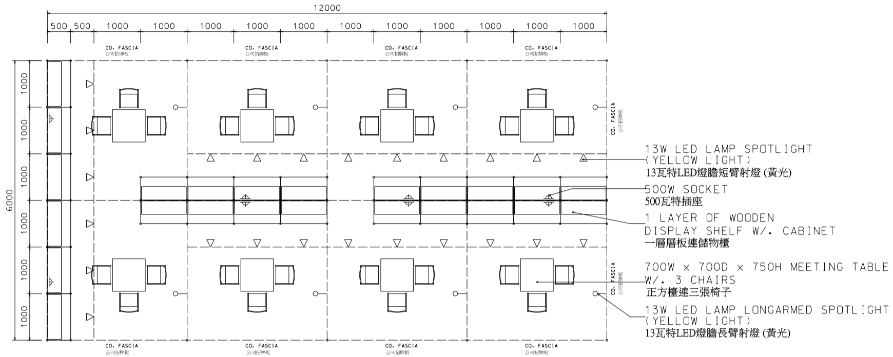
PLAN 平面圖
