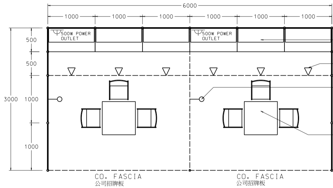
PLAN 平面圖
