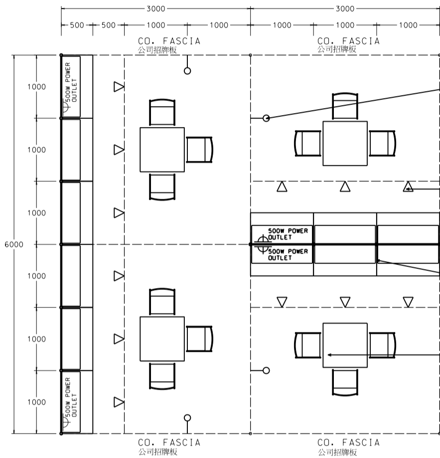
PLAN 平面圖
