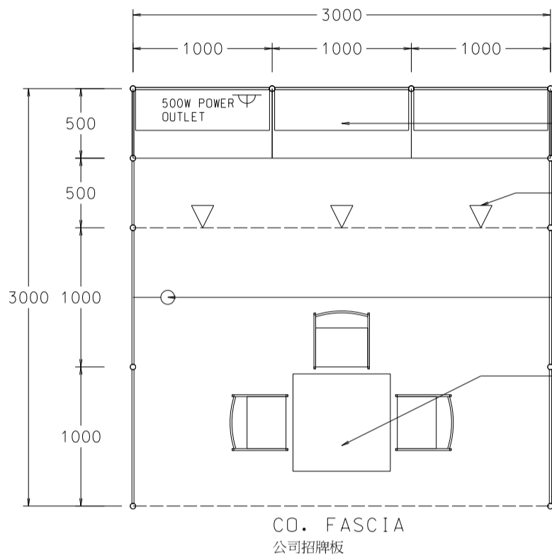
PLAN 平面圖
